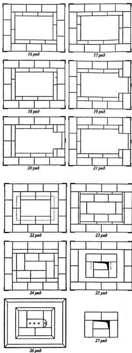
Рис. 5. Порядовка кладки банной печи-каменки № 1 (продолжение)
